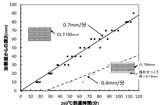
図 4 CLT パネルの炭化速度
