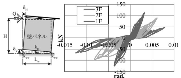
図 3 CLT 構造のモデル化と各層の荷重変形関係
