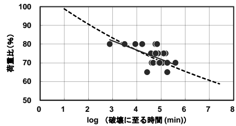
図 2 CLT がクリープ破壊に至る時間
