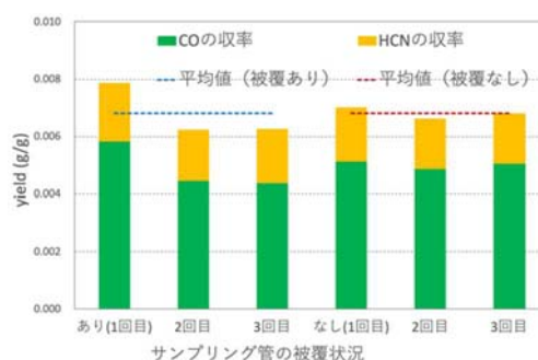
図5 サンプリング管の被覆有無の比較
