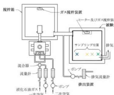
図 1 ガス有害性試験装置の概略図
