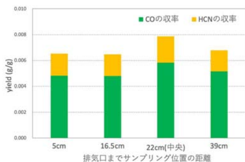
図3 サンプリング位置の比較
