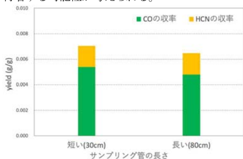
図4 サンプリング管の長さの比較
