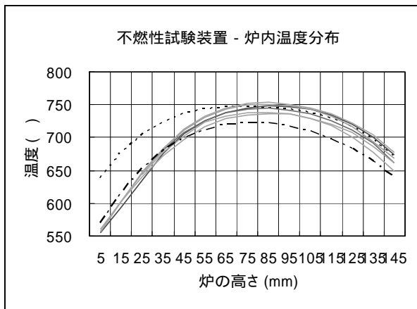
図 - 1 炉内温度分布(各試験機関)
