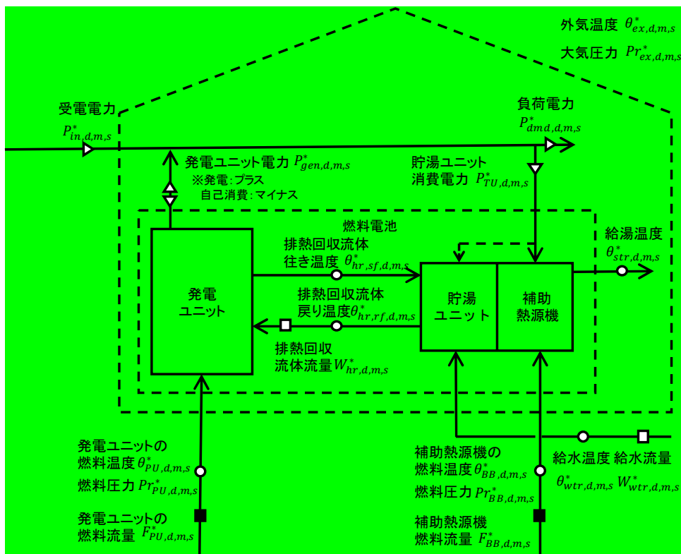
図 3.3 燃料電池試験におけるデータ測定箇所
