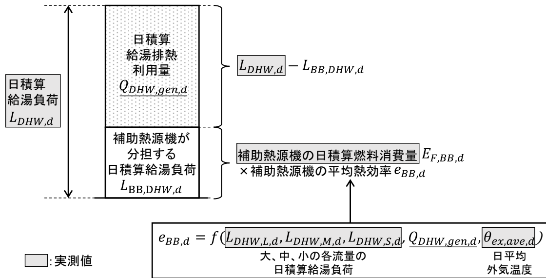
図 6.14 日積算給湯排熱利用量 Q_{DHW,gen,d} の概念図
